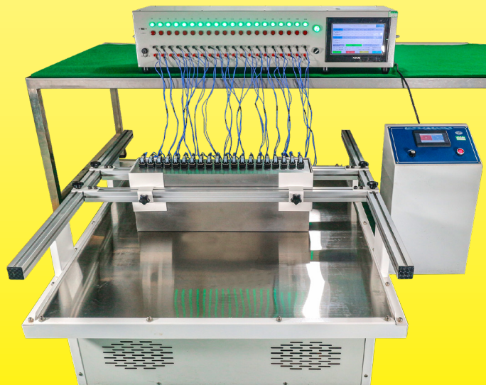
Apparecchiatura di test per misurare la resistenza alle vibrazioni degli interruttori pneumatici e il contatto a lenta azione dei pressostati mediante simulazione delle condizioni di trasporto (Laboratorio Ultimheat)
